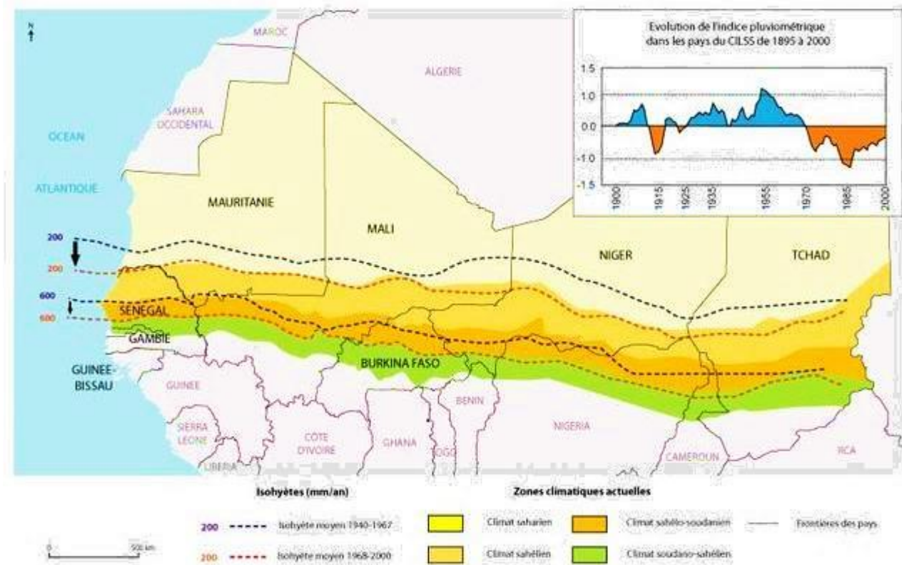
Figure 28: Rainfall and Climate Zones in West Africa (source : Club du Sahel et de l'Afrique de l'Ouest, 2007)
