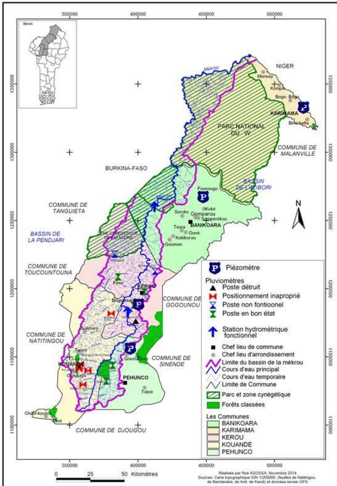
Carte 8 : Equipements de production de données sur l'eau dans le bassin de la Mékrou
